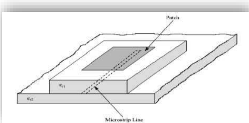
Gambar 3.1 Geometri patch antenna mikrostrip dengan teknik pencatuan electro-magnetically coupled
